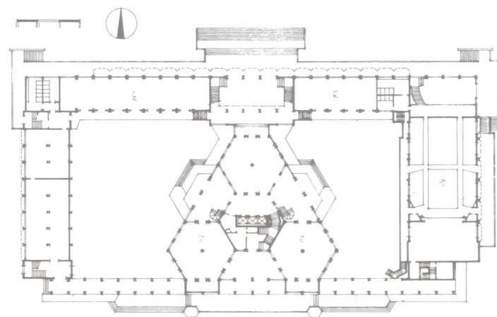
■ 工人文化宫底层平面图
