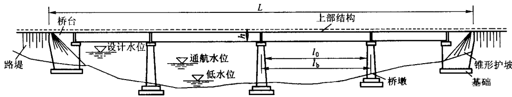
图 1-1-1 梁式桥
