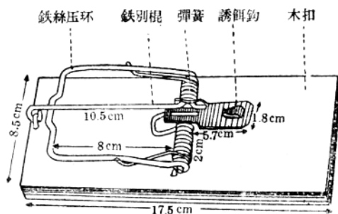
图 10 甲 木板鼠夹
