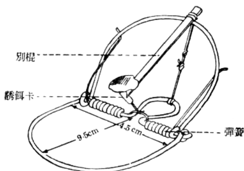
圖 11 針絲鼠夾
