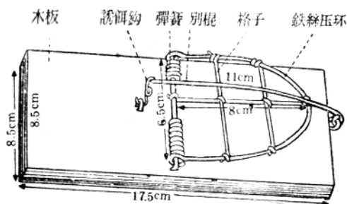
圖 10 乙 木板鼠夾
