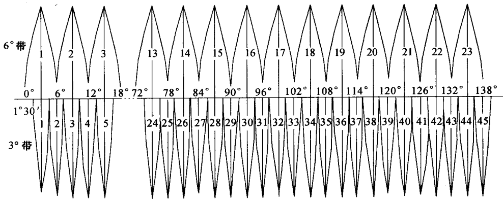
图 1-5 高斯投影 6^\circ 带与 3^\circ 带
