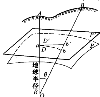
图 1-9 水平面代替水准面
