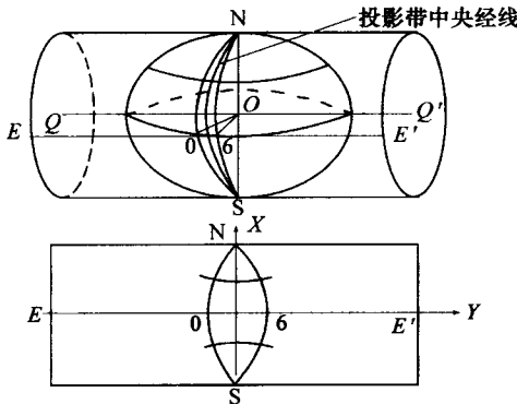
图 1-6 高斯投影的特点
