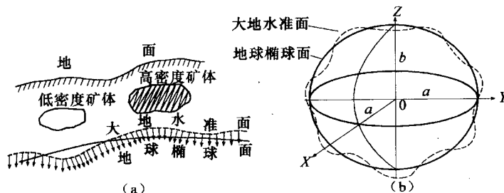
图 1-1 大地水准面与地球椭球面
