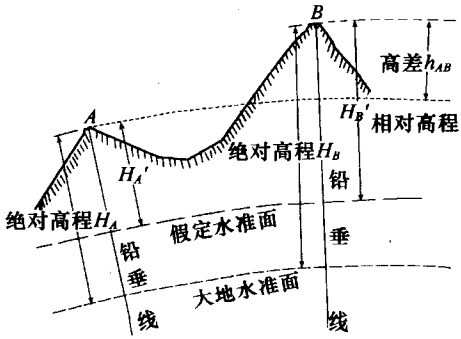
图 1-8 绝对高程与相对高程
