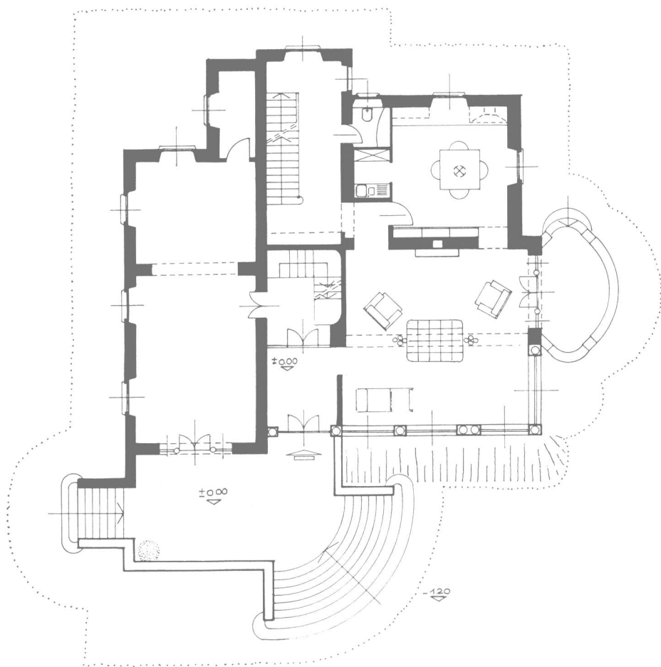
一层平面图
