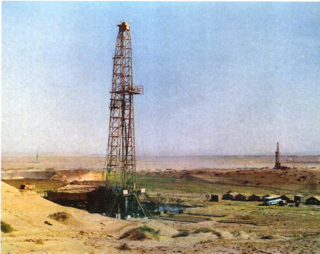
南疆石油勘探区
