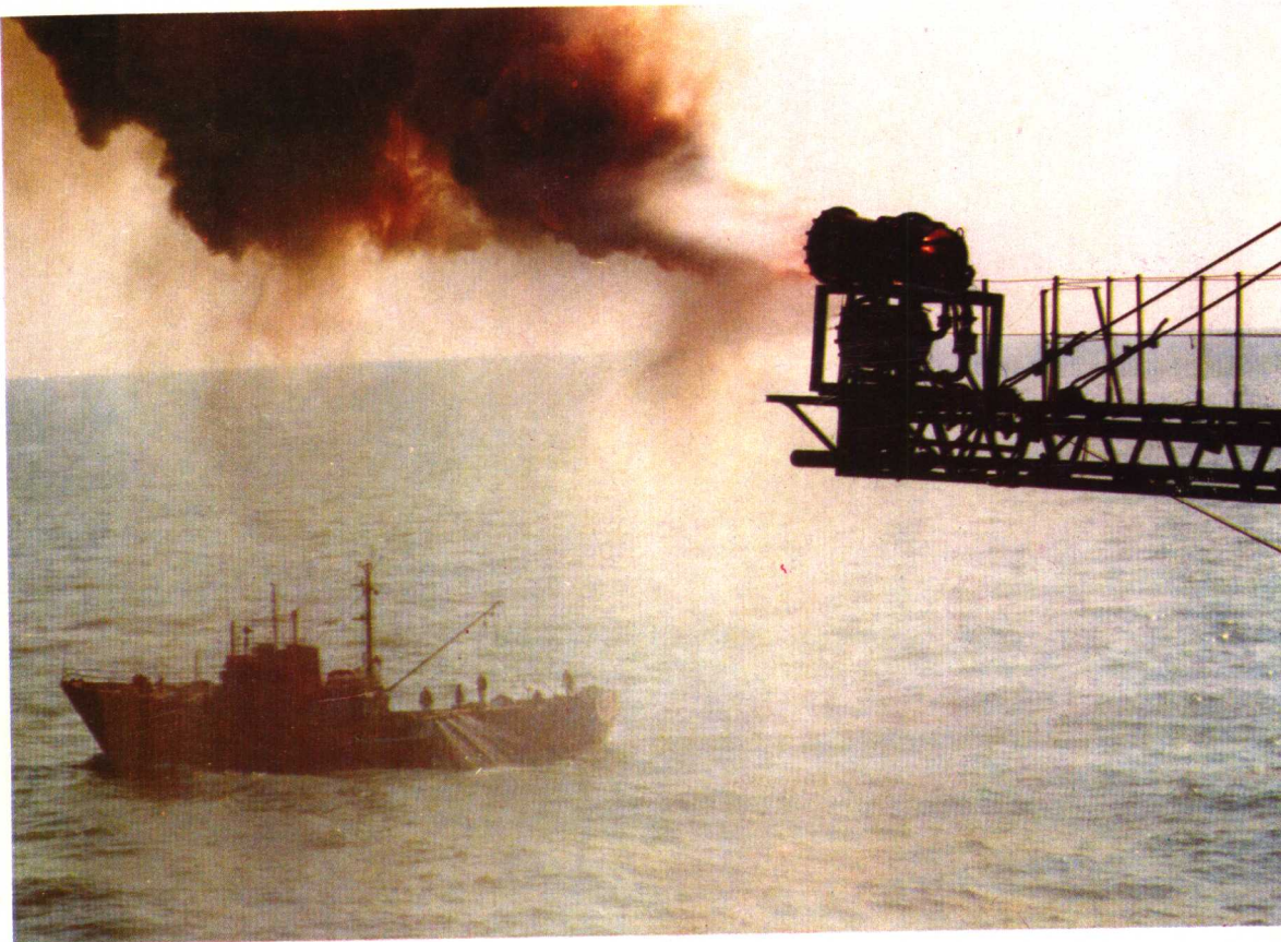
南海石油勘探区
