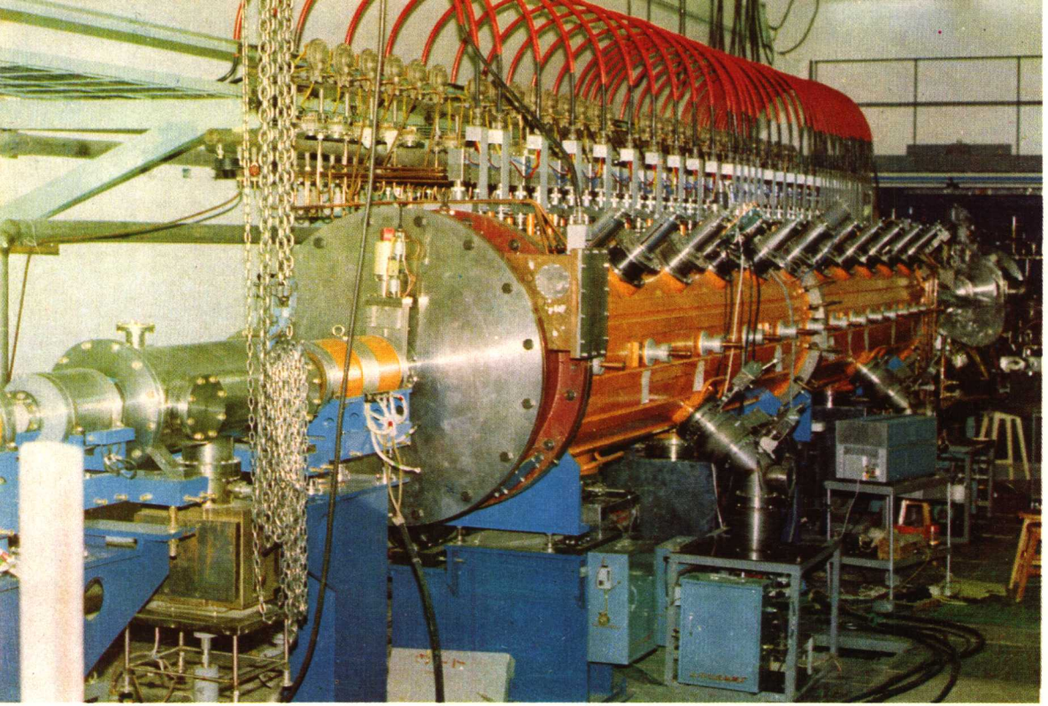
我国第一台10兆电子伏特质子直线加速器
