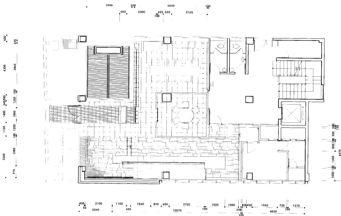
一层平面图
