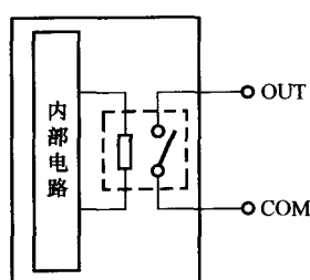
(a) 继电器输出型
