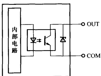
(b) 晶体管输出型
