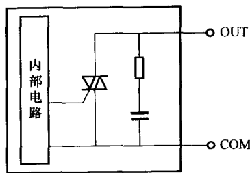
(c) 晶闸管输出型
