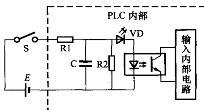
图 1.1.2 输入接口电路
