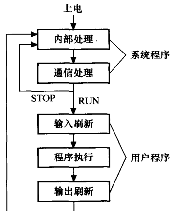
图 1.1.4 PLC 典型的扫描周期
