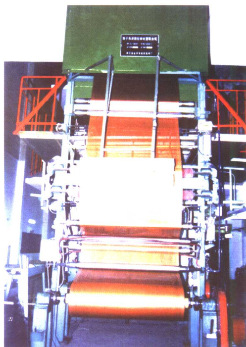
锦纶6浸胶帘子布浸胶机
