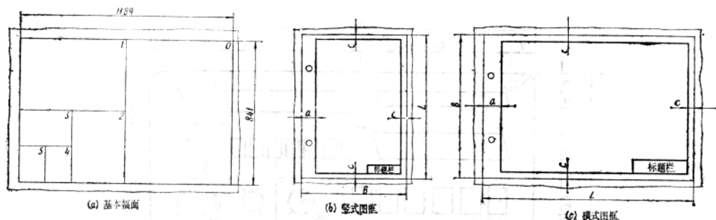
图 1-17 图幅
