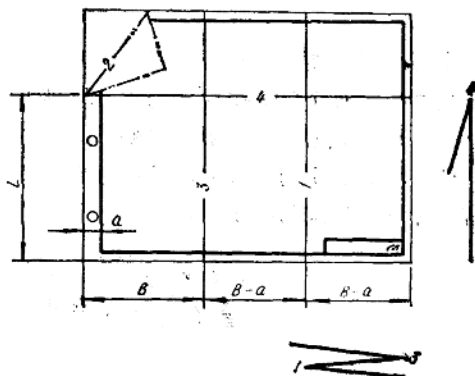
图 1—19 图纸折叠法
