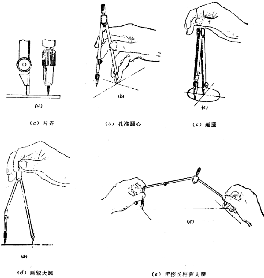
图 1—7 圆规的用法
