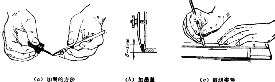
图 1—9 鸭咀笔的用法
