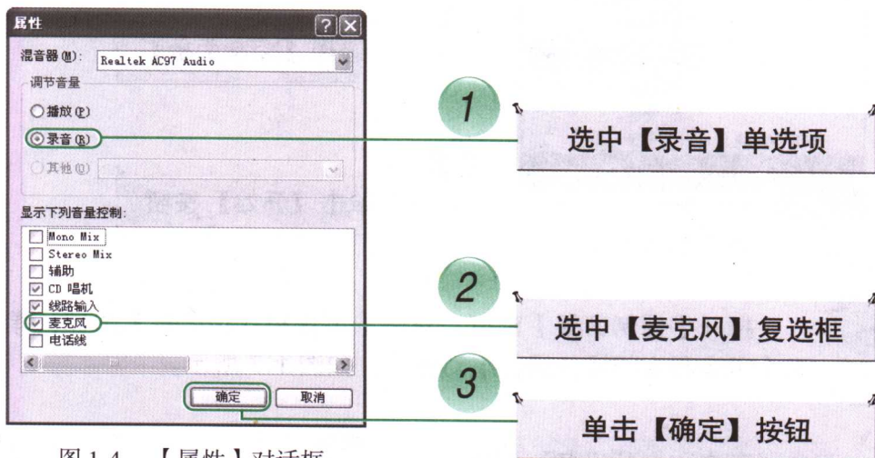
图 1.4 【属性】对话框
