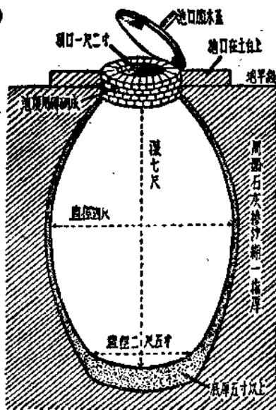
瓦甕式茅池(容量三十担)圖樣
