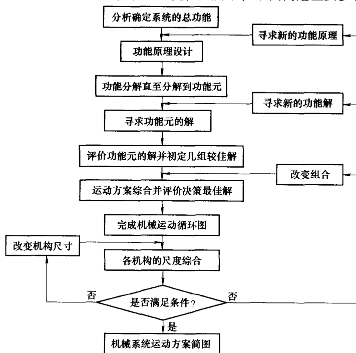
图 2-1 机械运动方案设计流程图
