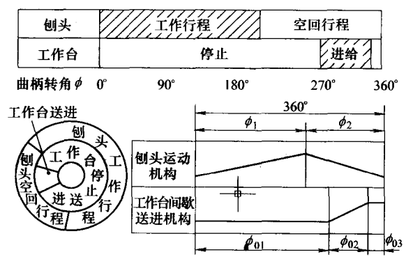
图 2-7 牛头刨床的运动循环图
