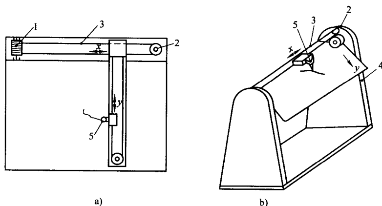
图 2-5 绘图机
