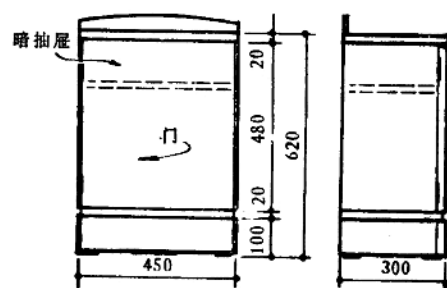
M 1:20 床边柜
