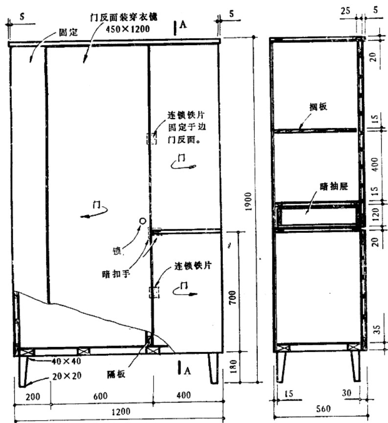
大衣柜 M 1:20
