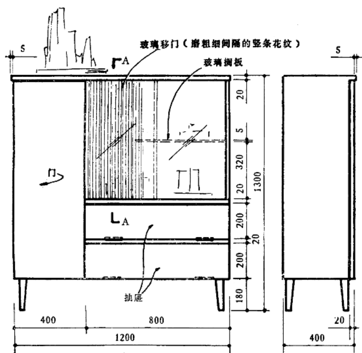
食品柜 M 1:20
