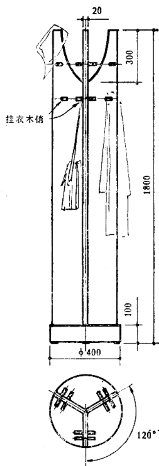
衣帽架 M 1:20
