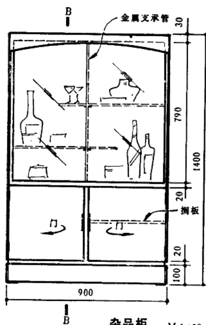
杂品柜
