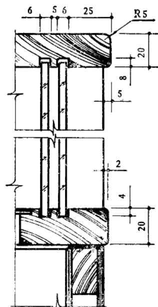
A-A 玻璃移门结构 M 1:2
