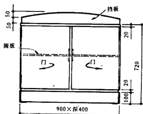
M 1:20 茶具柜
