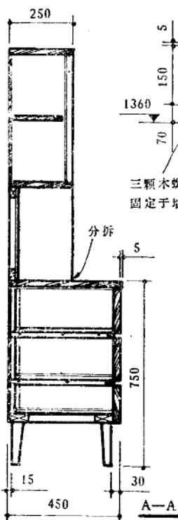
书柜 M1:20
