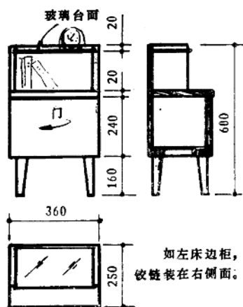
床边柜 (右) M 1:20
