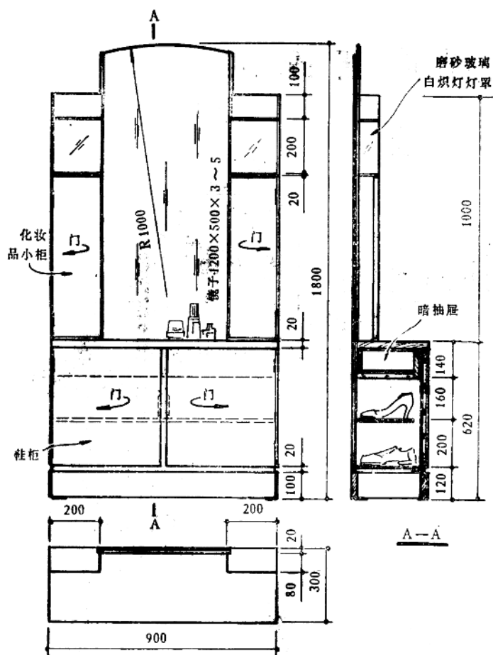
化妆桌 M 1:20
