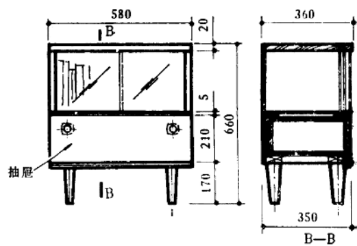
床头柜 M1:20
