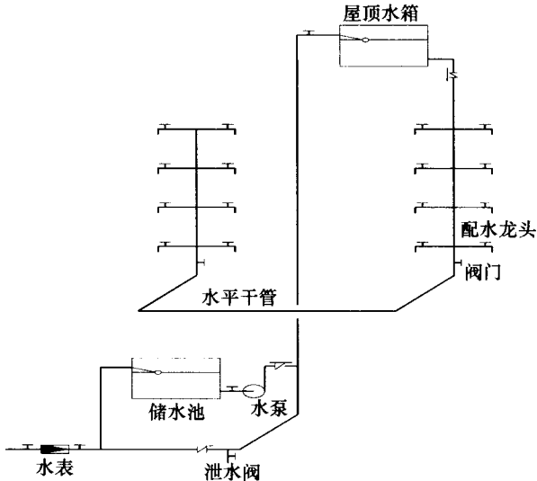
图 1-4 设水泵和水箱的给水方式
