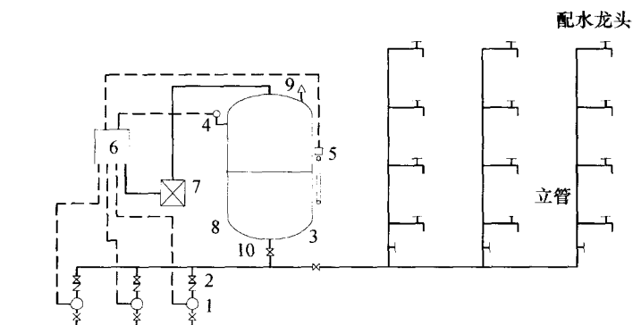
图 1-5 气压给水方式
