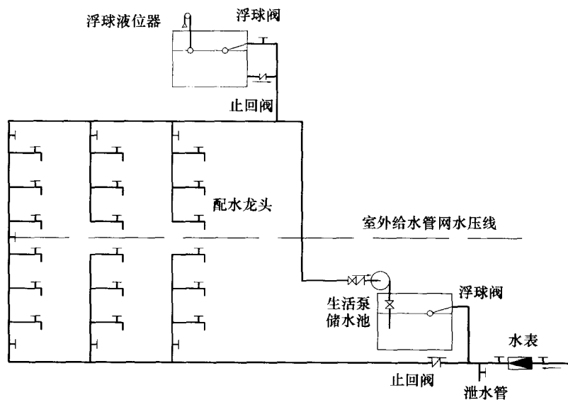
图 1-6 分区给水方式
