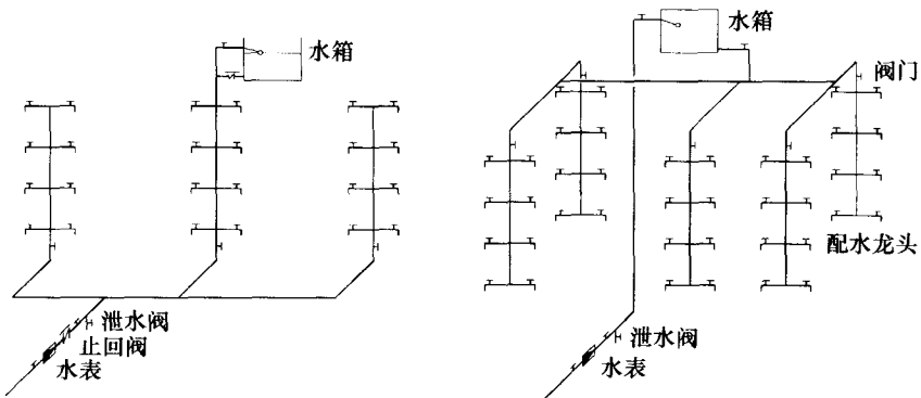
图 1-2 设水箱的给水方式
