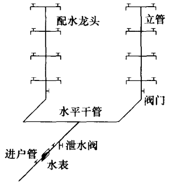
图 1-1 直接给水方式
