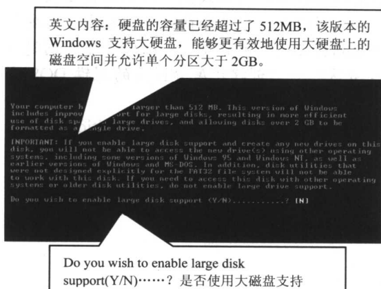
图 1-1 FDISK 命令
