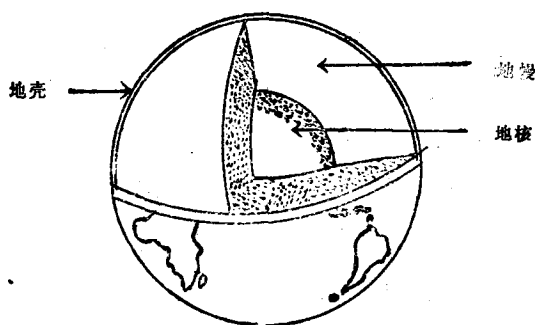
图一 地球内部的构造
