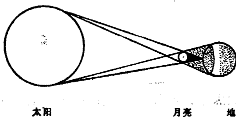
图二 日食示意图
