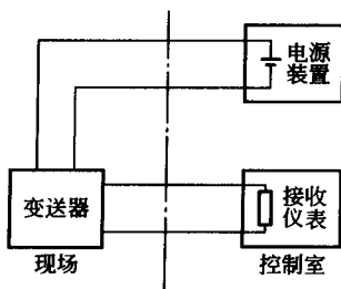
图 0-4 四线制传输
