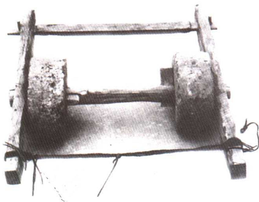
图 20 二轮砣子(出自河北)。石砣直径 28 厘米,厚 11 厘米,框架长 76 厘米,宽 70 厘米。出处同上。
