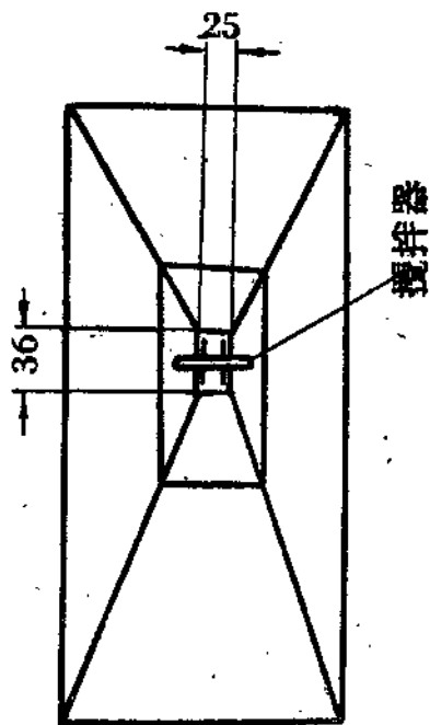
种子箱俯视图
