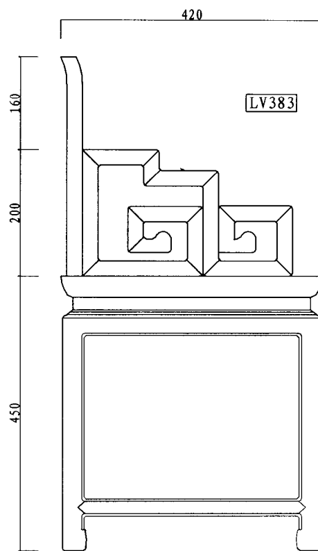
左视图 left view
