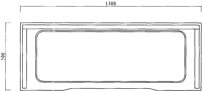
俯视图 top view
