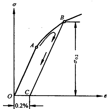
图 1-2 \sigma_{0.2} 的确定
