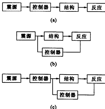
图 1.3 主动控制形式或类型
