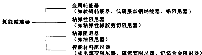
图 1.6 耗能减震器按耗能材料分类
