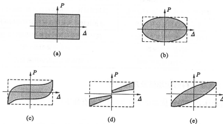
图 1.9 不同阻尼器的滞回曲线形状
