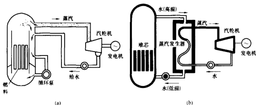
图 1-4 核电厂生产过程示意图 (a) 沸水堆型反应堆；(b) 压水堆型反应堆
