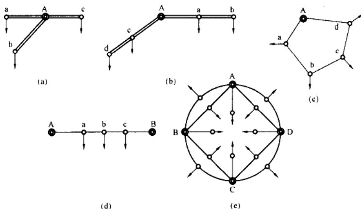
图 1-6 有备用接线形式
