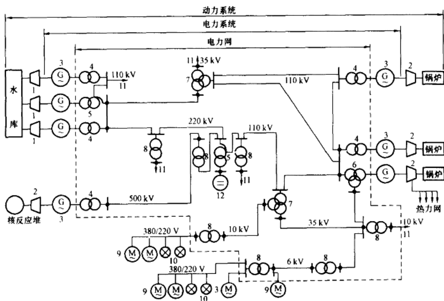
图 1-1 动力系统、电力系统、电力网的示意图
