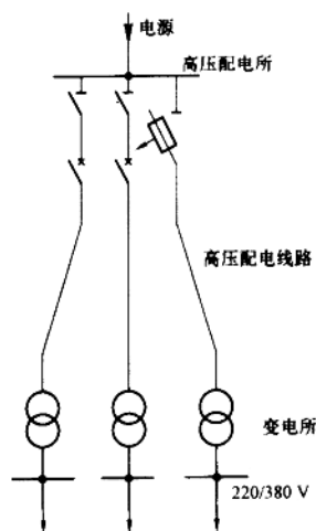
图 1-7 放射式网络
