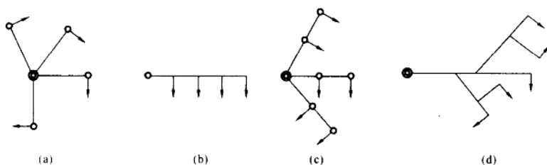
图 1-5 无备用接线形式
