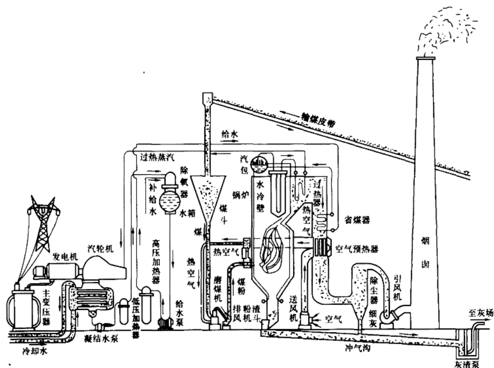
图 1-2 火电厂生产过程示意图
