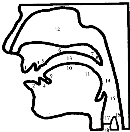
图一 发音器官示意图
