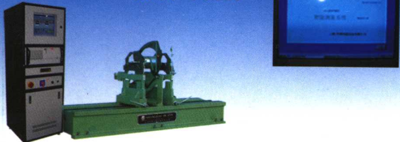
YYQ硬支承平衡机
