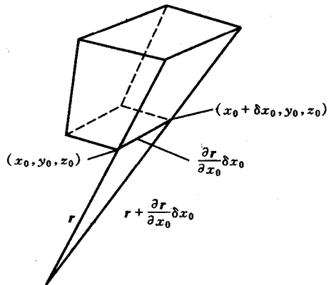
图 1.1 拉格朗日坐标系中的流体微元
