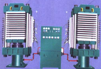
▲塑料地板成型机 SLC-Q 1050 \times 1050 \times 12/3.0MN SLC-Q 760 \times 1000 \times 10/2.5MN SLC-Q 1400 \times 10/0.5MN
