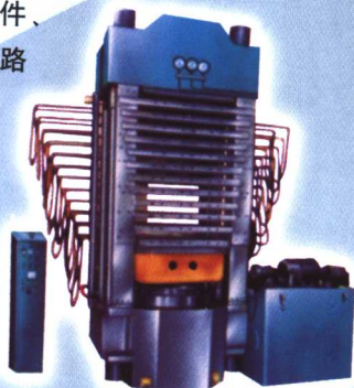
XLB-Q/D125×300~1500×2000 400t~1500t平板硫化机
