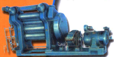
橡胶三、四辊压延机
