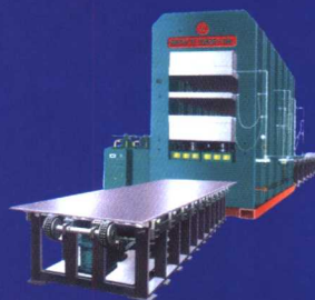
▲XLB-Q1400 \times 6200 \times 2/34 MN 履带平板硫化机
