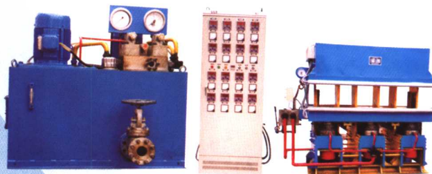
XLE-D350×2000~350×4000 双面颚式平板硫化机
