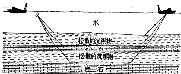
图7 用地震法勘探海底构造
