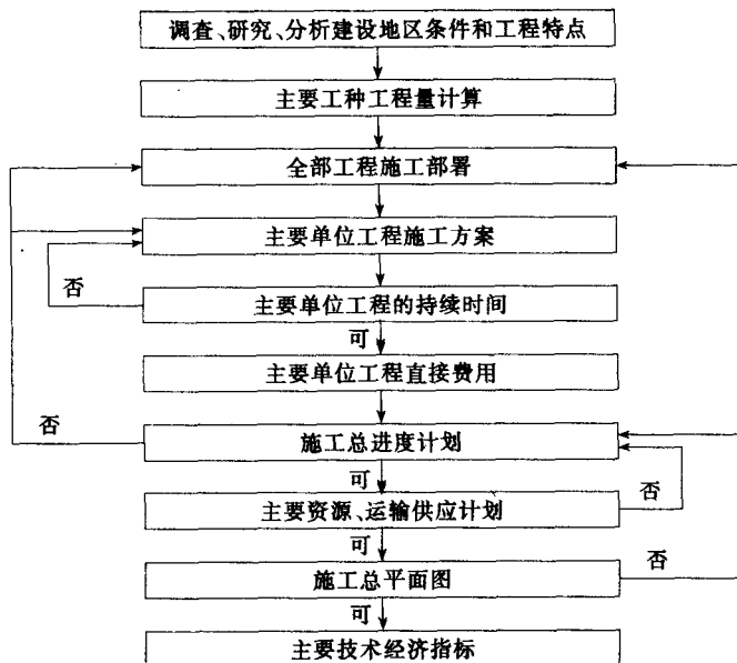
图 1-1 施工组织总设计编制程序
