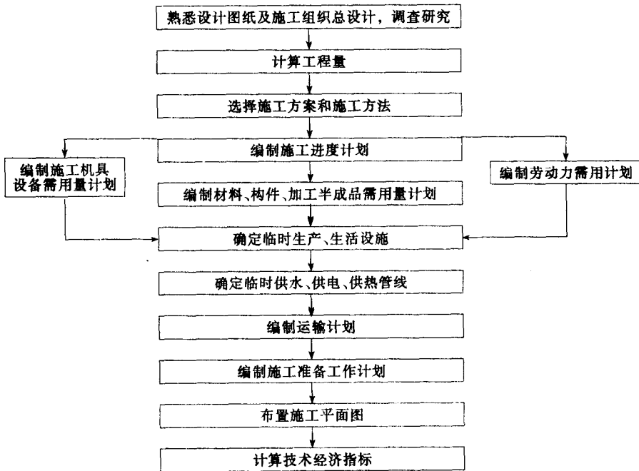
图 1-2 单位工程施工组织设计编制程序
