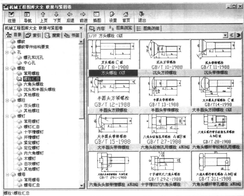
图 2-1 软件界面
