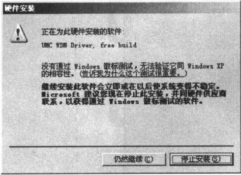
图 1-11 系统提示
