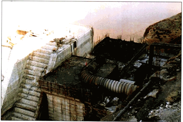
左岸引黄取水 口施工现场
