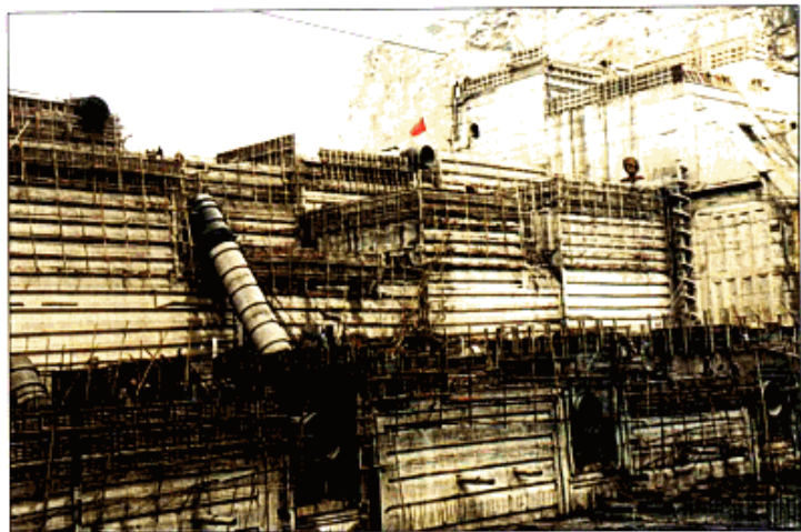
排砂钢管安装现场
