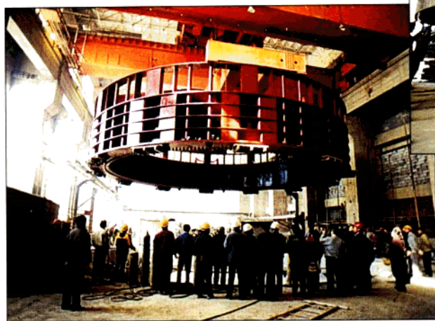
定子吊装
