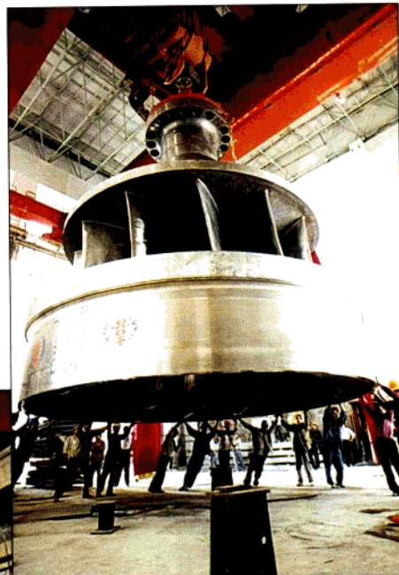
转轮吊装
