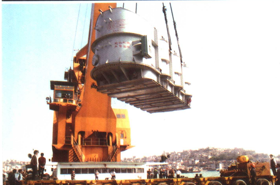
22万伏输电变电设备运抵石狮
