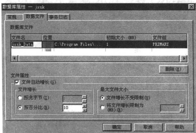
图 1-5 数据库 jxsk 属性中数据文件选项卡
