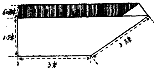
第三圖 藥浴池的構造圖
