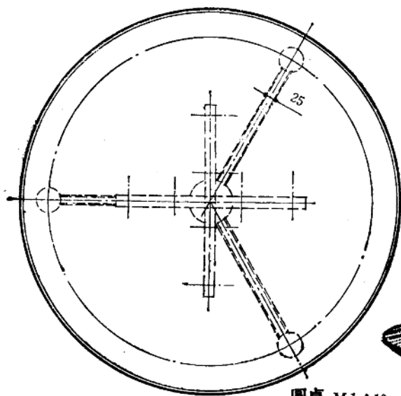
圆凳 M1:10
