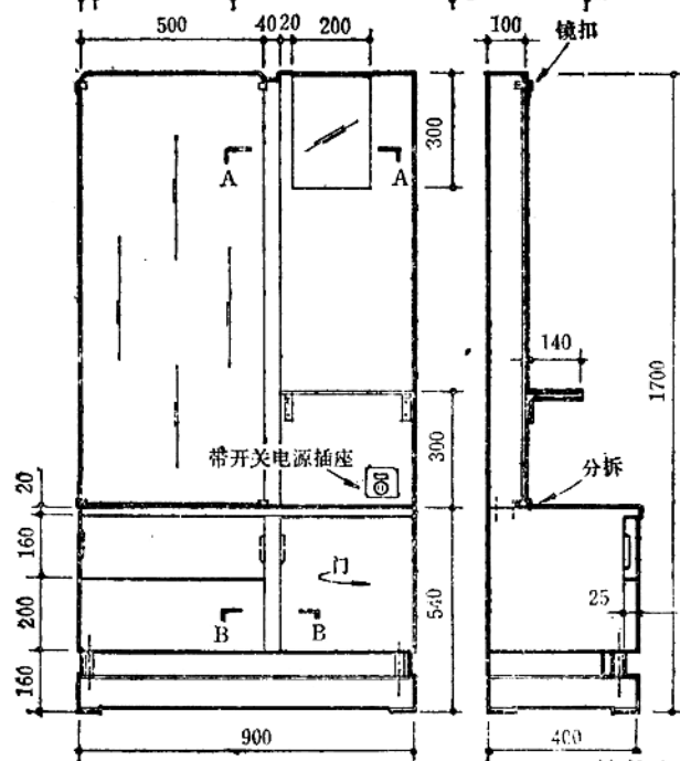
梳妆桌 M1:20
