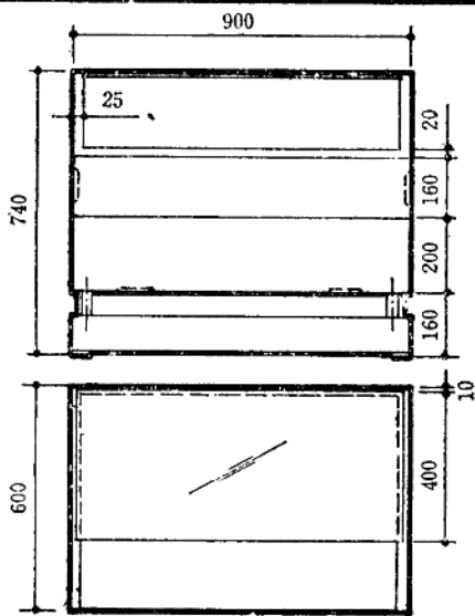
陈设柜 M1:20
