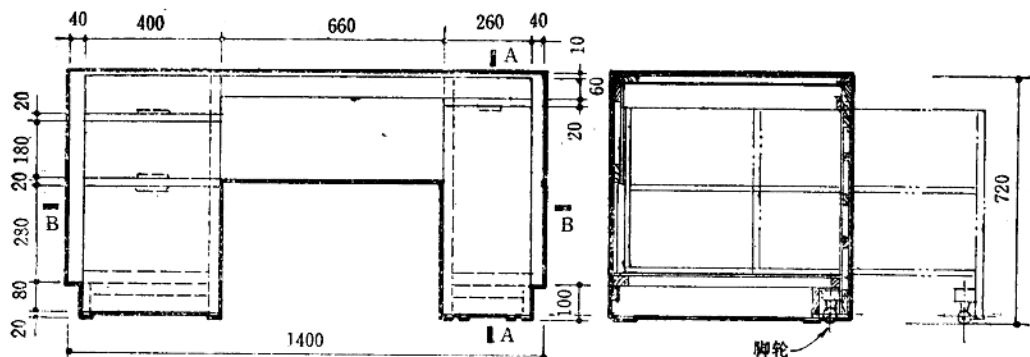
写字桌 M1:20
