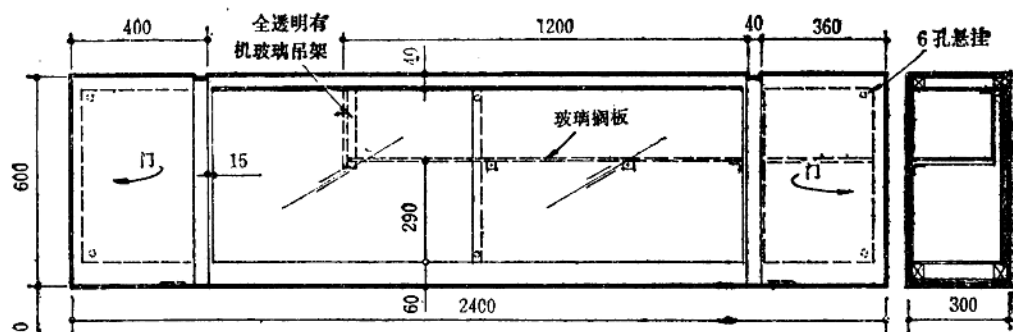
悬挂书架 M1:20
