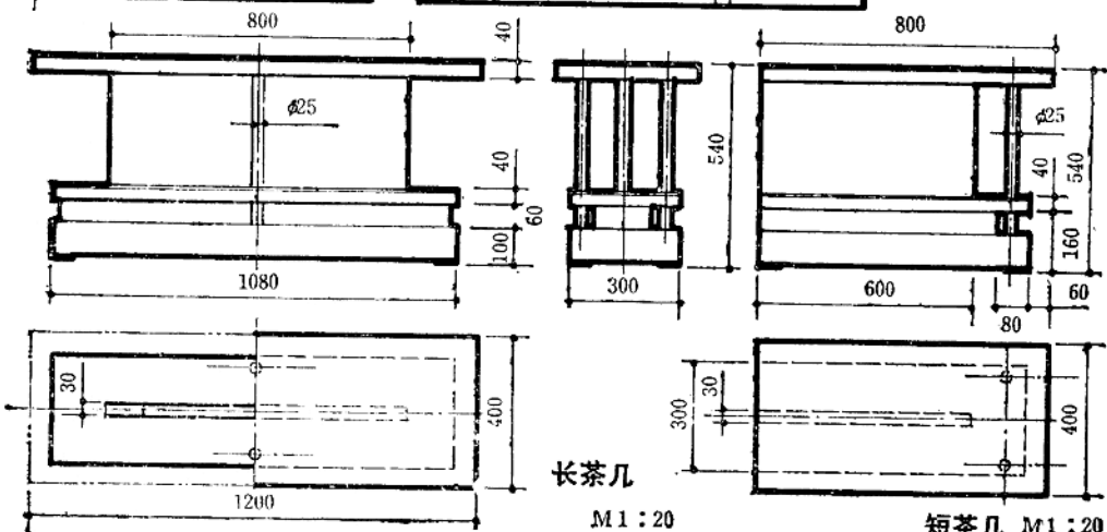
短茶几 M1 : 20
