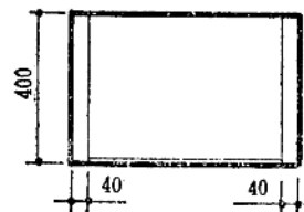
低柜 M1:20
