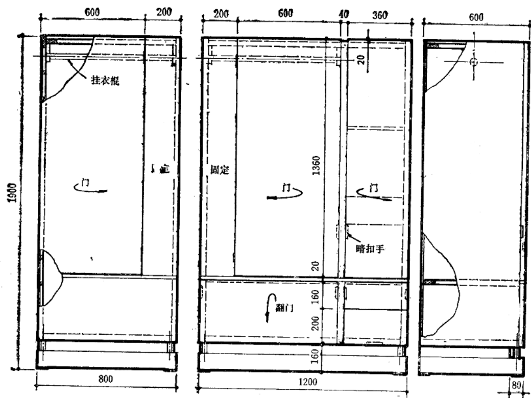
挂衣柜 A 挂衣柜 B
