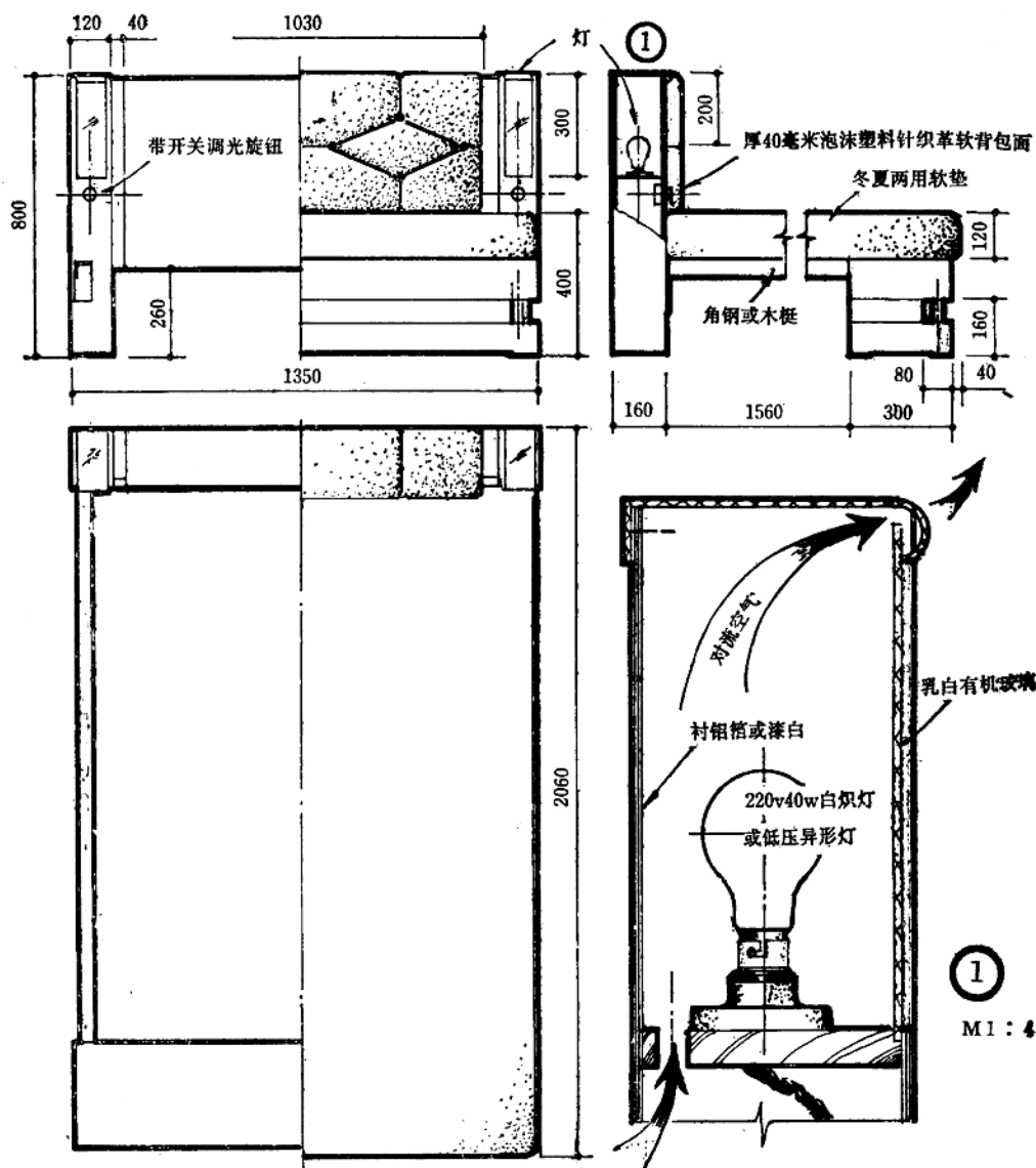
带灯双人床 M1:20
