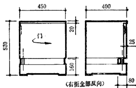
左床边柜 M1:20
