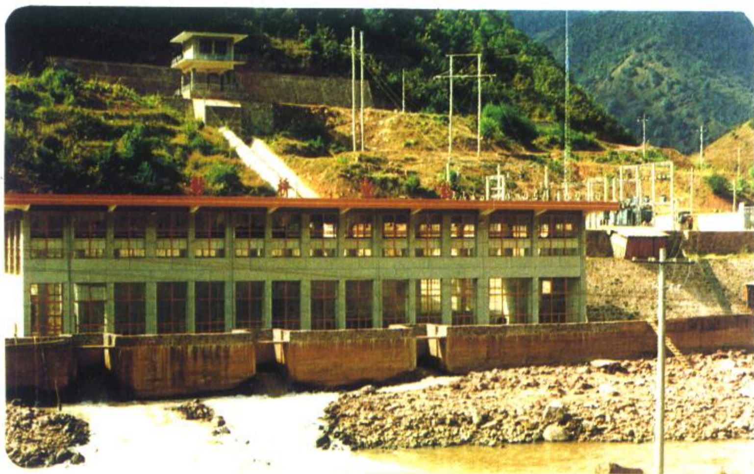
装机容量为二千四百千瓦的新桥电站
