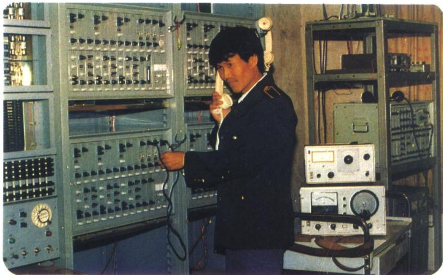
邮电局十二路环路载波机在工作
