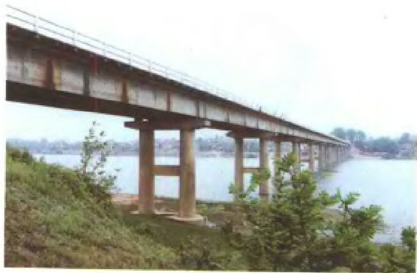
▶ 座落于余干县黄埠镇的黄 金埠大桥，上部为钢筋混 凝土装配式预应力丁梁， 下部为薄壁沉井，钢筋混 凝土基础
