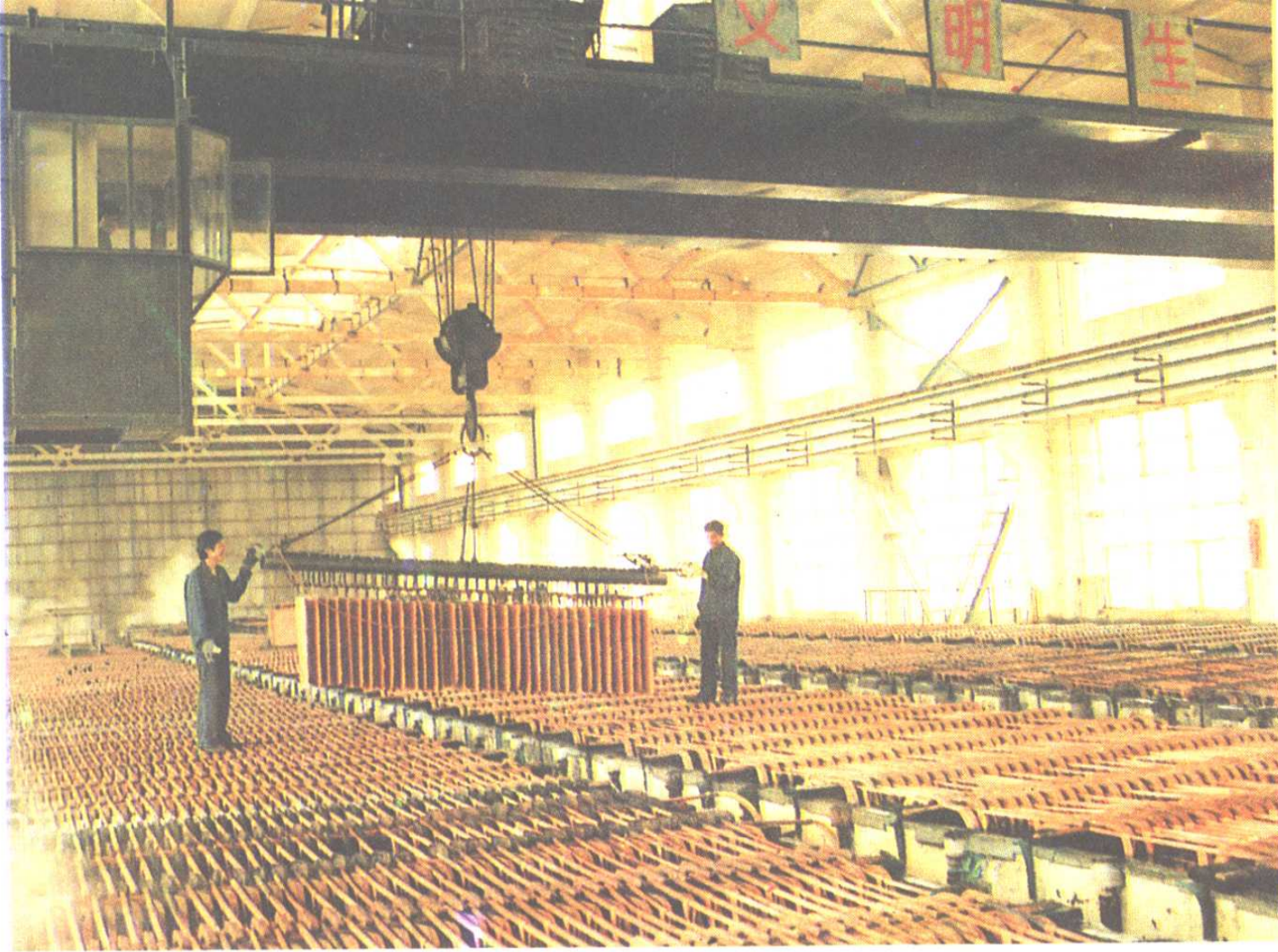
电解铜车间
