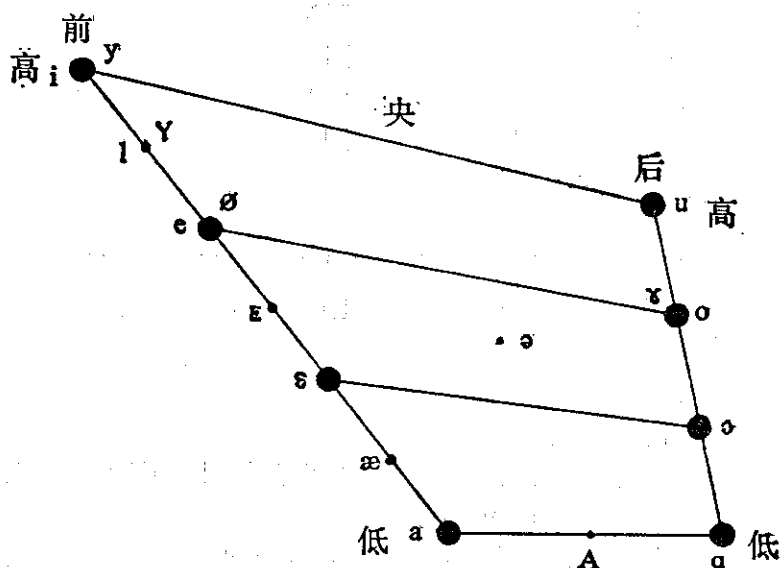
元 音 图
