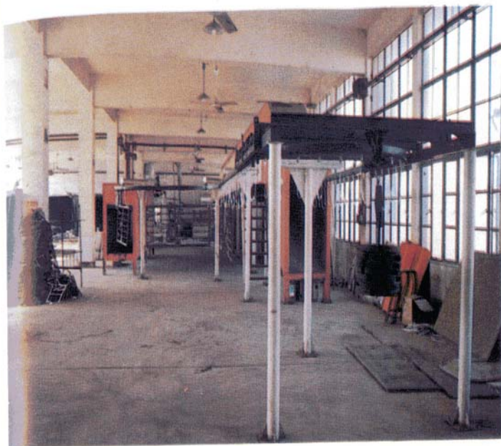
南京金属家具总厂塑料喷涂生产线
