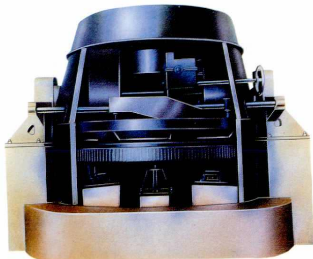
φ1600 × 450 湿式轮碾机
