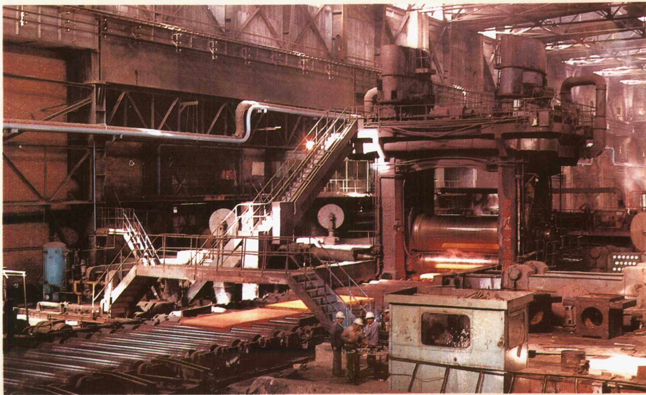
舞阳钢铁公司4200毫米轧钢机
