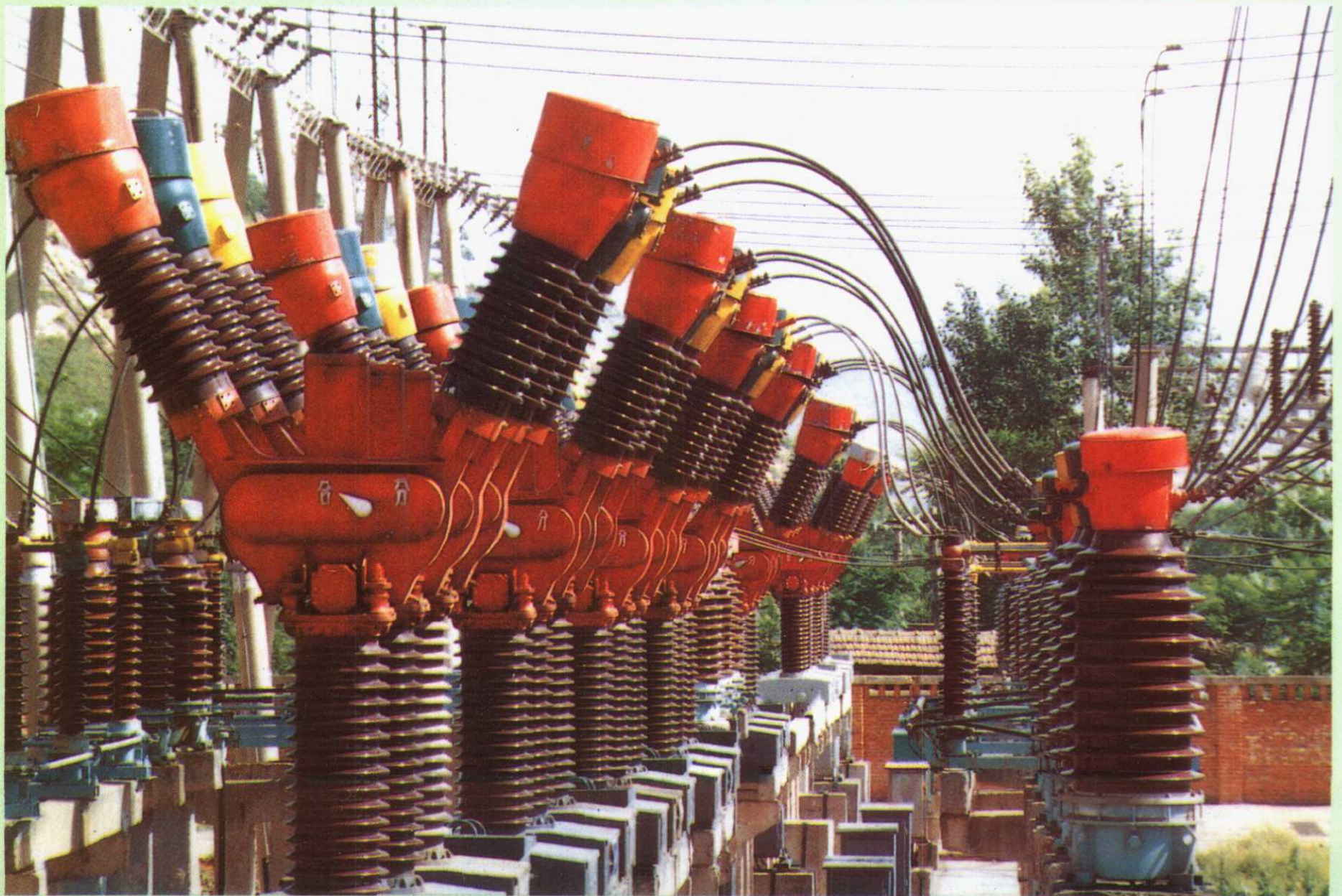
小石门 22 万伏变电站
