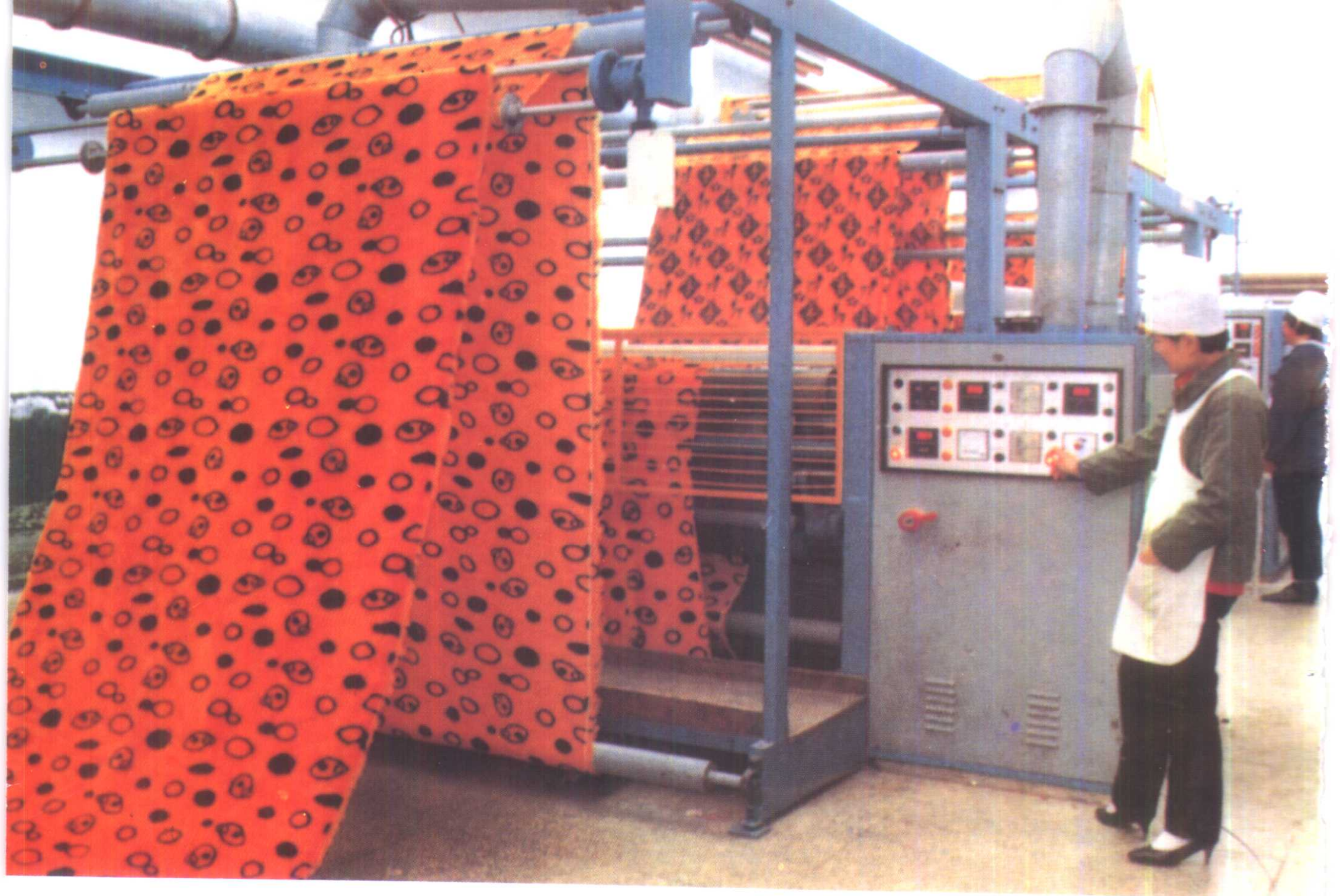
人造毛皮厂生产车间
