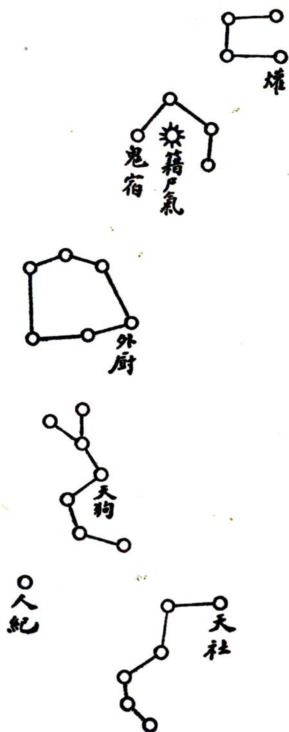
鬼宿全圖
