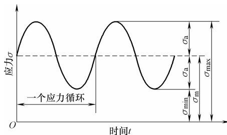
图 1-1 应力循环
