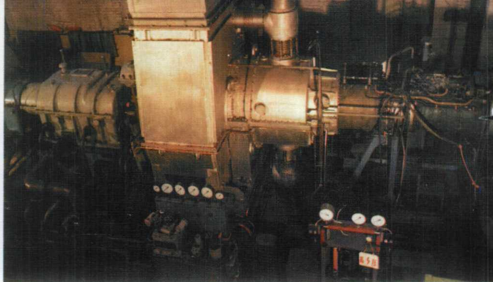
▶ 航空工业部黎明机械公司制造的 WP 6G 1A 燃汽轮 机热电并供机组 (航空工业部供稿)
