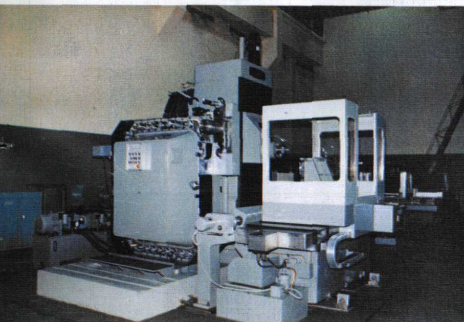
◀ 昆明机床厂生产 的我国自行设计的第一 台THK 4680精密 全闭环卧式加工中心
