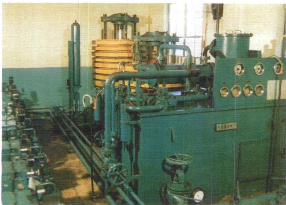
▶ 大连液压件厂研制 的线材轧机大型成套液 压系统
