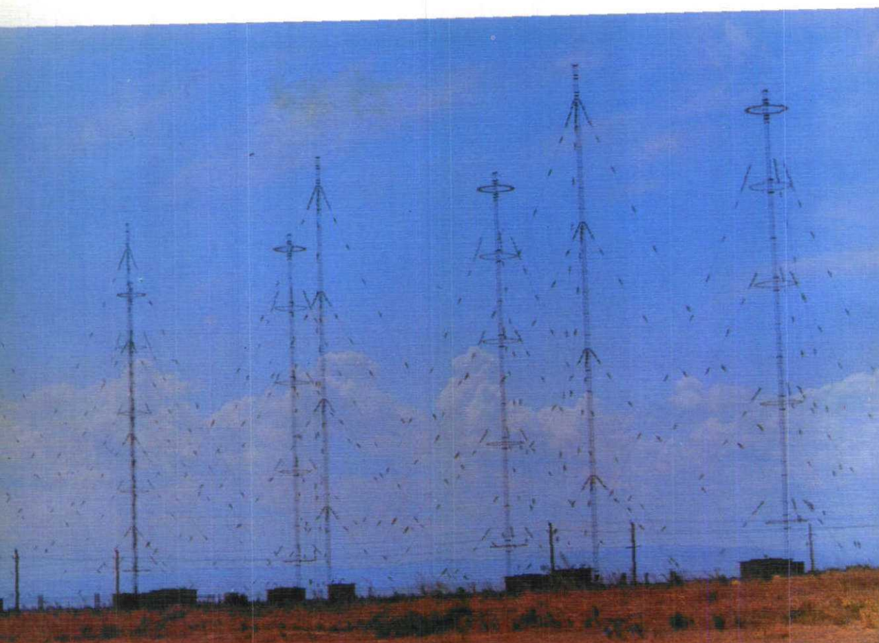
▼ 我国建成的2000KW天线阵
