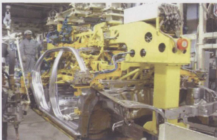
模夹一体化产品——侧围线
