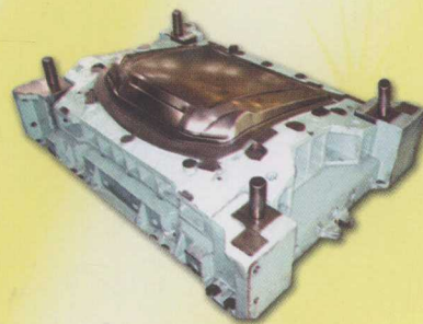
发动机罩外板拉延模
