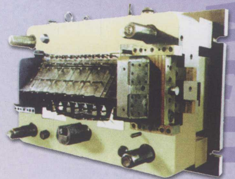
整体梯级压铸模
